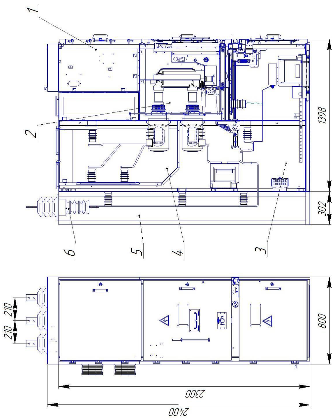
1-релейный шкаф ; 2-отсек выключателя ; 3-отсек линейных шин и кабельных соединений; 4-отсек сборных шин; 5-короб шинного ввода; 6-проходной изолятор
