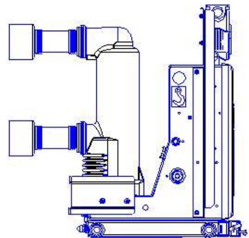
выкатной элемент с вакуумным выключателем VF12 (EVOLIS, SHELL, BB/TEL, Sion)
