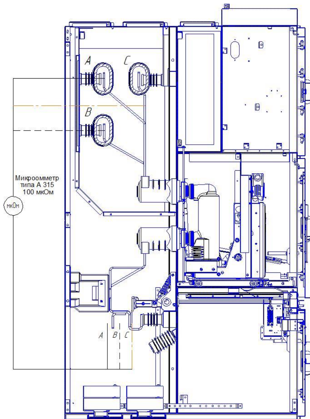
Рисунок Б.21 - Схема измерения омических сопротивлений фаз методом сравнения с эталонным сопротивлением.
