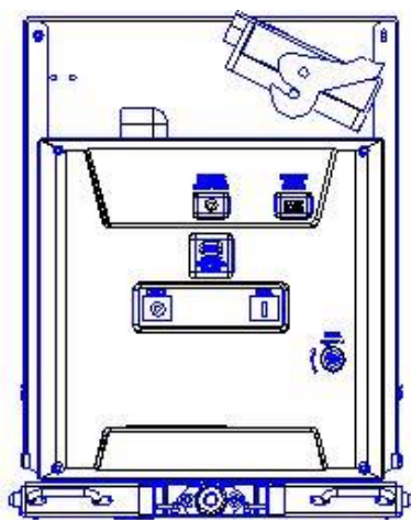
выкатной элемент с вакуумным выключателем VF12 (EVOLIS, SHELL, BB/TEL, Sion)
