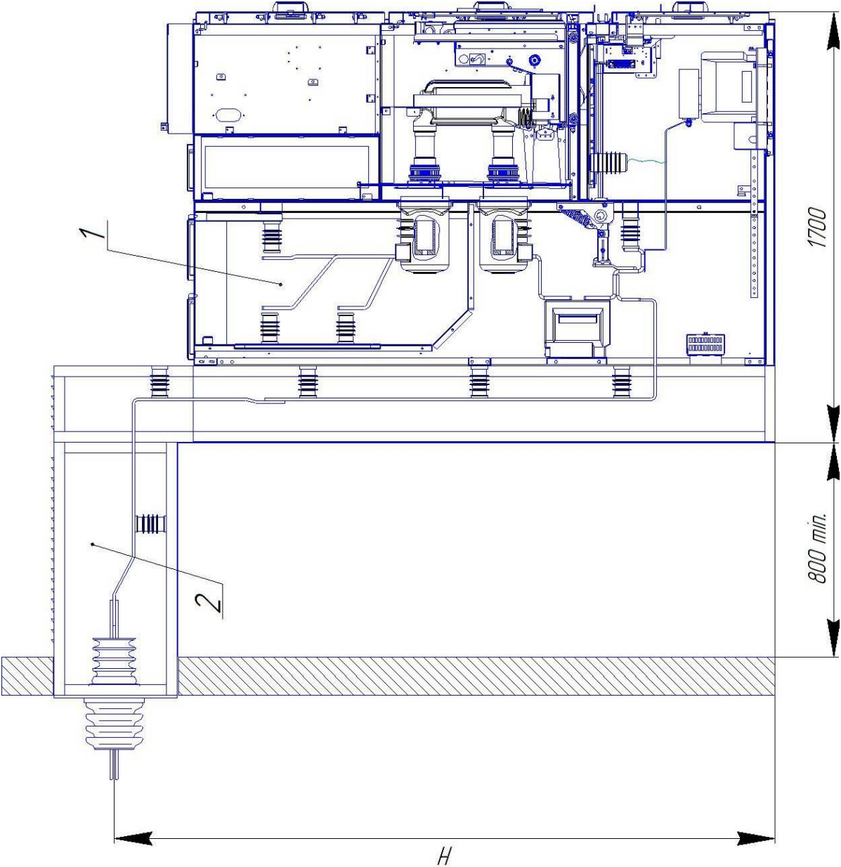
Рисунок Б.16 - Компоновка шинного ввода (размеры L и H определяются проектом или заказчиком)
